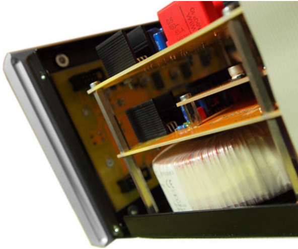
Die Energieversorgung verantwortet ein 100-VA-Ringkerntrafo. Entscheidender als schiere Leistung seien aber die Maßnahmen zur Spannungsstabilisierung, so Norma, die man bei den HS-DA1-Geräten sehr aufwändig konzipiert habe
